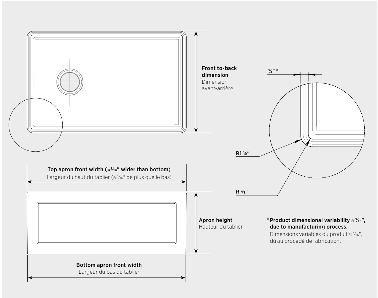
IMAGE 5 SINK INSTALLATION / INSTALLATION DE L'ÉVIER
