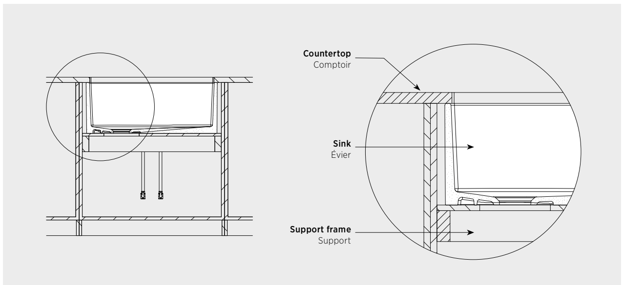
IMAGE 5 SINK INSTALLATION / INSTALLATION DE L'ÉVIER
