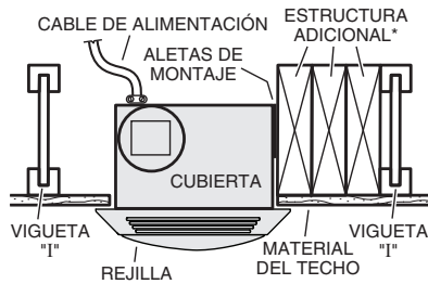
CUBIERTA MONTADA EN CUALQUIER LUGAR ENTRE LAS VIGUETAS Se requiere una estructura adicional para las aletas de montaje.
