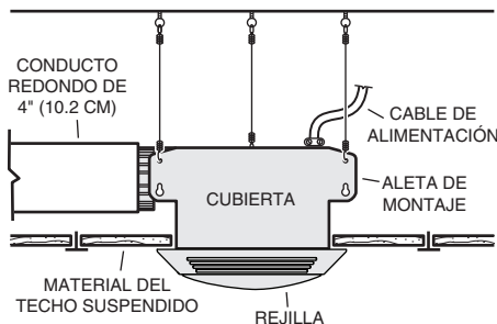
TECHOS SUSPENDIDOS Cubierto montada con cables. Montaje de tres puntos.
